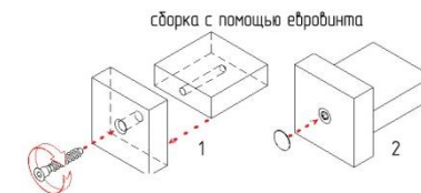
сборка с помощью евровинта
