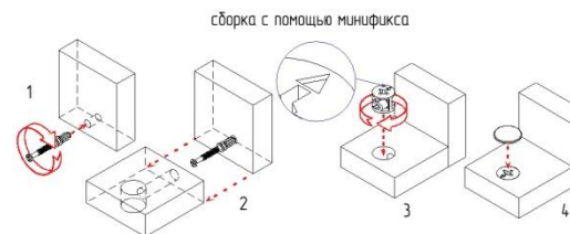
сборка с помощью минификса
