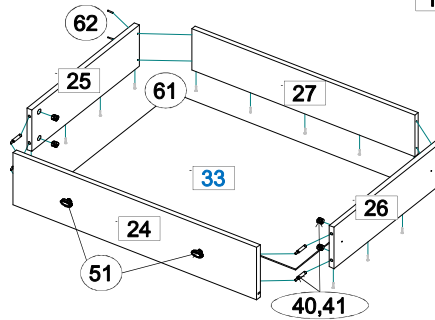
Эксцентриковая стяжка
