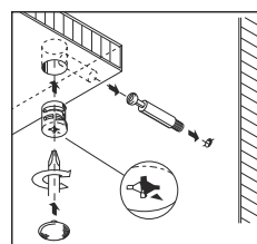
Монтаж эксцентриковой стяжки
