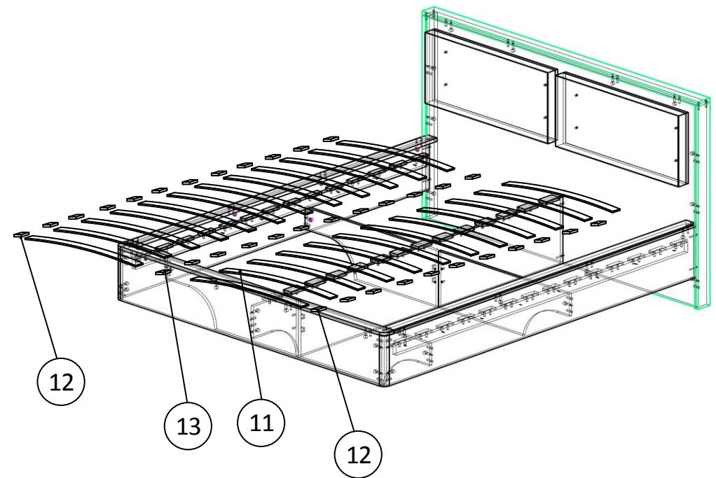
Рисунок 4 – Установка лат
