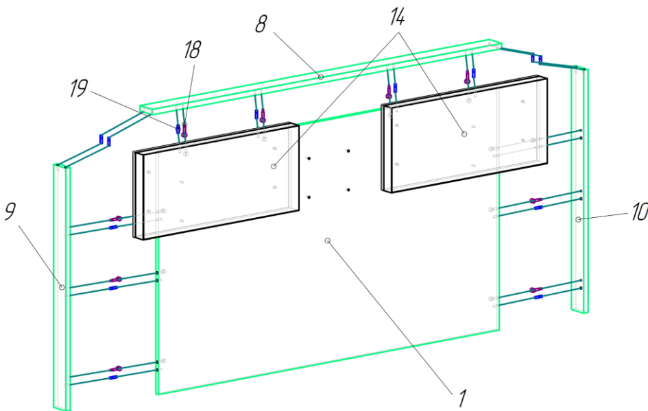
Рисунок 1 – Сборка щита
