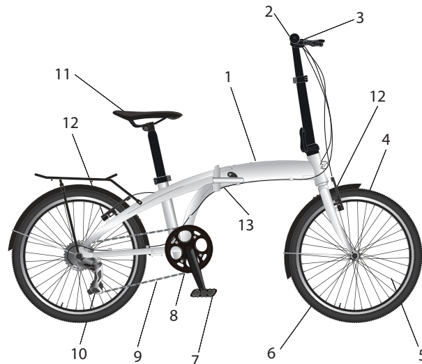
Схема складного велосипеда со складным рулем
