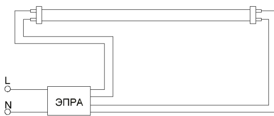
Светильник с ЭПРА до замены
