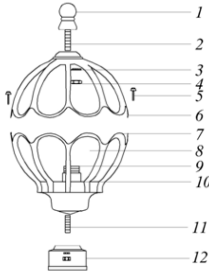
1 – балясина; 2 – резьбовое крепление; 3 – гровер; 4 – гайка; 5 – винты; 6 – верхняя крышка; 7 – нижняя крышка; 8 – рассеиватель; 9 – патрон; 10 – ламподдержатель; 11 – резьбовое крепление; 12 – основание.
