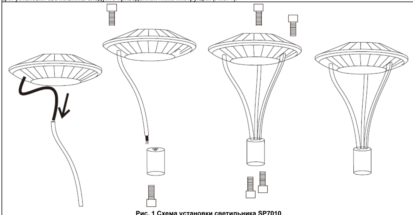
Рис. 1 Схема установки светильника SP7010
