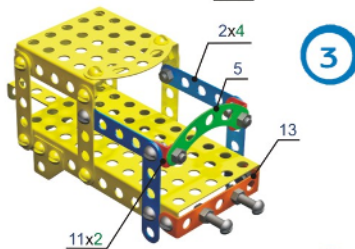
Пассажирский вагон
