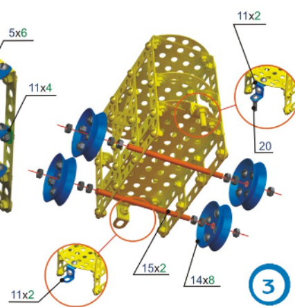
Пассажирский вагон
