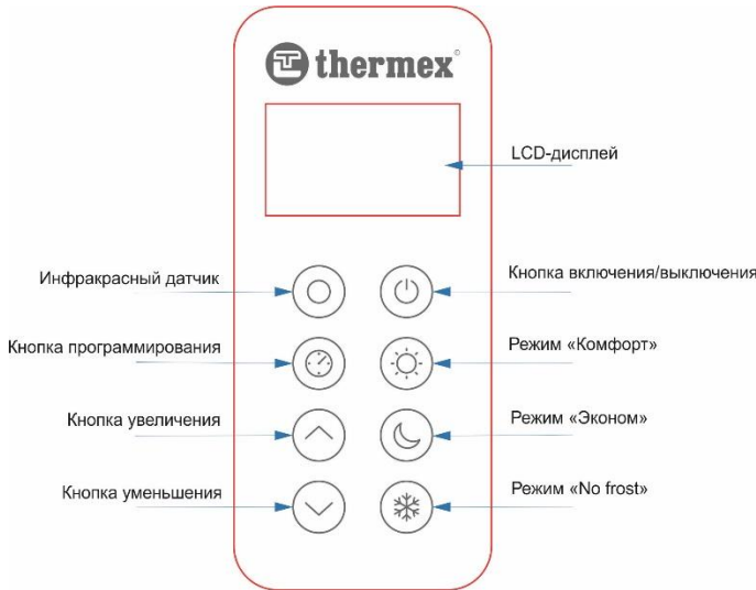
Рис. 5 Панель управления
