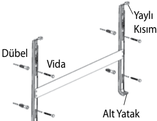
Şekil 5. Askı Kancaları
