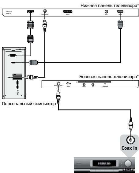
Усилитель
