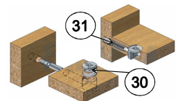
Эксцентриковая стяжка
