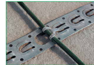
▲ Крепление кабеля к ленте
