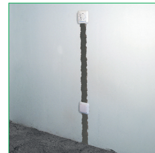
Штробы заделывают после заливки секций раствором и проверки отсутствия повреждений
