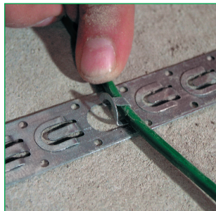
▲ Крепление кабеля к ленте
