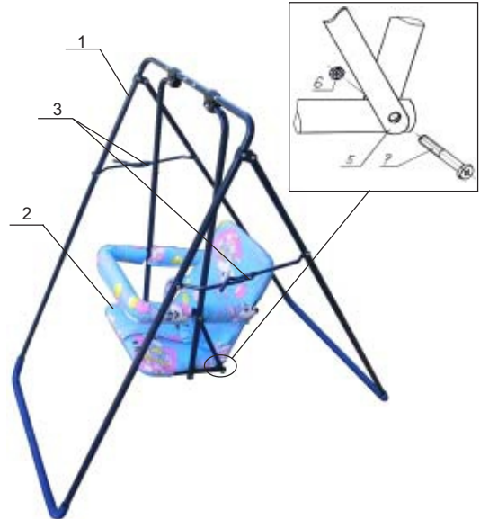
Рисунок 2. Сборка качелей
