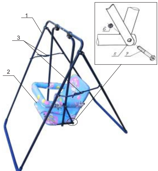
Рисунок 2. Сборка качелей
