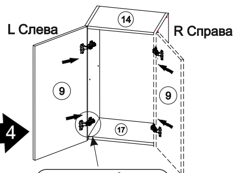
Варианты установки фасада
