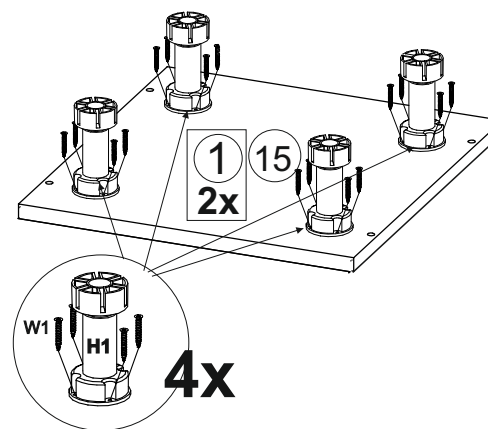
Установка регулируемых опор
