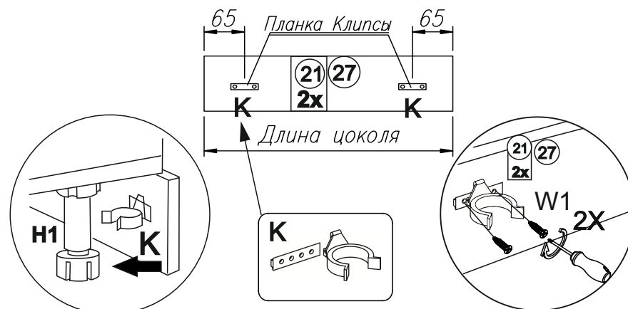
Установка цоколя
