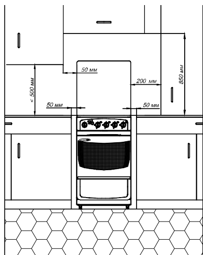
Рисунок 6 – Схема установки плиты
