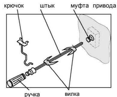
Рисунок 11 – Схема установки вертела
