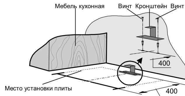
Рисунок 8 – Порядок установки кронштейна
