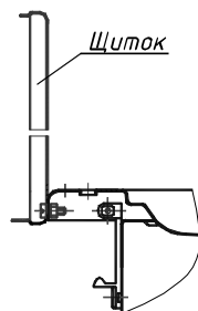
Рисунок 7 – Крепление щитка
