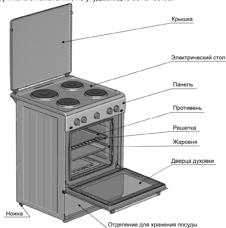
Рисунок 1 – Устройство плиты
