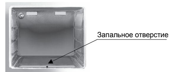
Рисунок 11 – Зажигание горелки духовки
