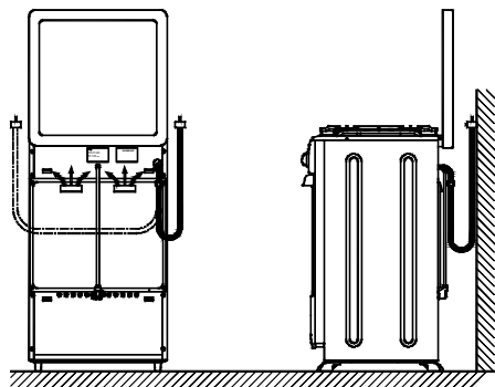
Рисунок 10 – Примеры подключения шланга
