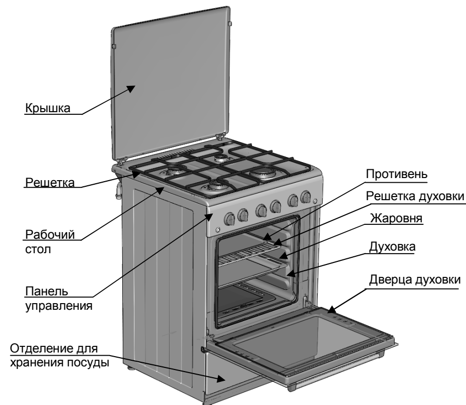
Рисунок 1 – Устройство плиты
