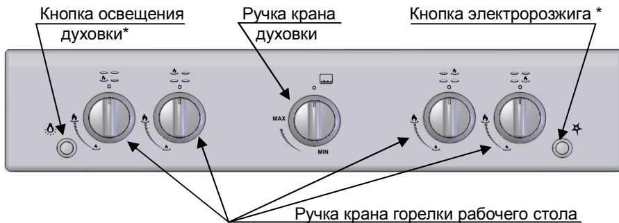
Рисунок 3 – Панель управления
