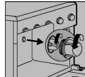
Рисунок 13 – Замена лампы освещения
