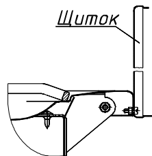
Рисунок 6 – Крепление щитка
