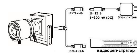
Схема подключения камеры.
