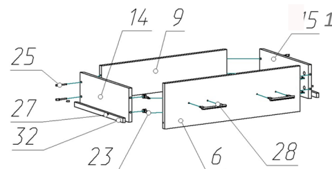
Рис.2 Сборка ящиков
