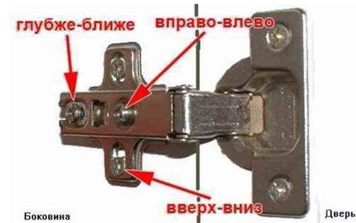
Рис.5 Крепление и регулировка распашного фасада
