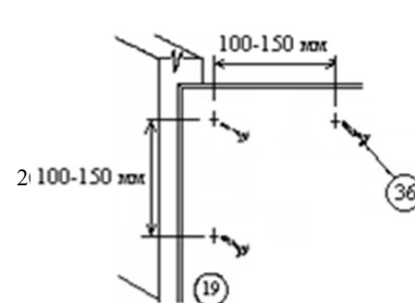
Рис.4 Крепление задней стенки и дна ящика
