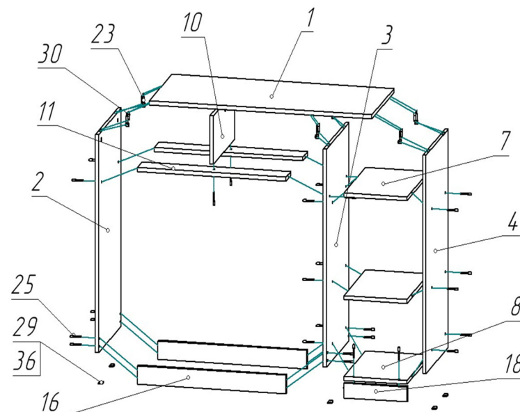
Рис.1 Сборка корпуса
