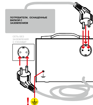
Схема подключения стабилизатора в сеть без заземляющего провода, с УЗО
