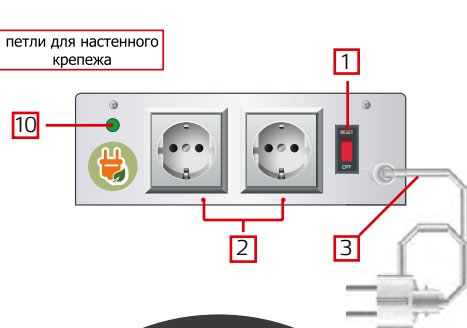
Нижняя панель
