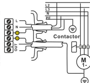
Схема подключения насосов с трехфазным сечением жил, напряжением 380 В, через пульт дистанционного управления.
