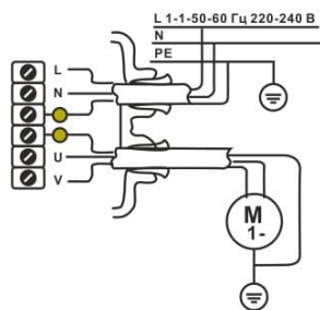
Схема подключения насосов с однофазным сечением жил, напряжением 230 В. и мощностью до 1,1 кВт.
