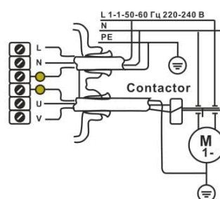
Схема подключения насосов с однофазным сечением жил, напряжением 230 В. и мощностью более 1,1 кВт., через пульт дистанционного управления.
