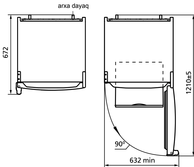
Şəkil 2 – Dondurucu (üstəndən görünüşü)
