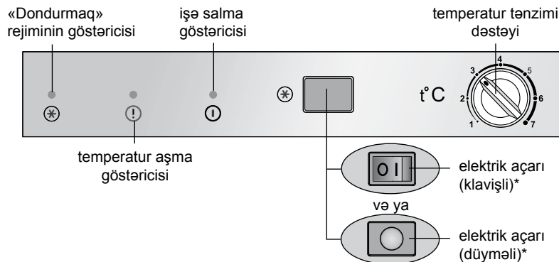
Şəkil 2 – Dondurucu (üstəndən görünüşü)
