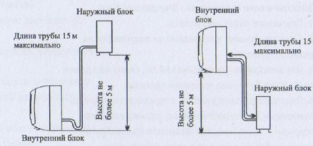
Схема установки
