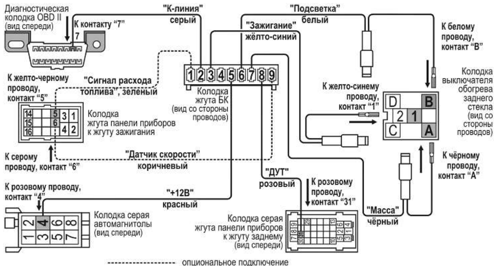
Рис.5 Схема подключения
