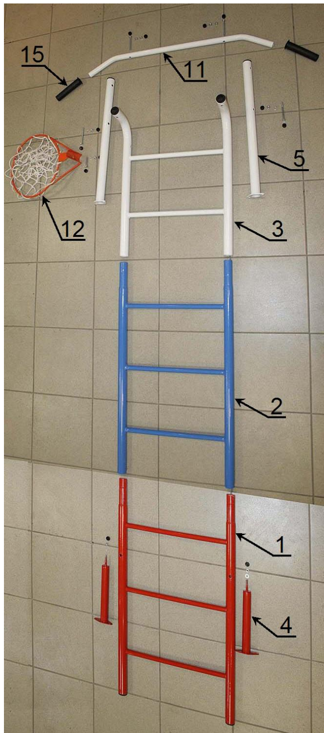
Рис.1. Сборочные единицы СК-15 «Чемпион»
