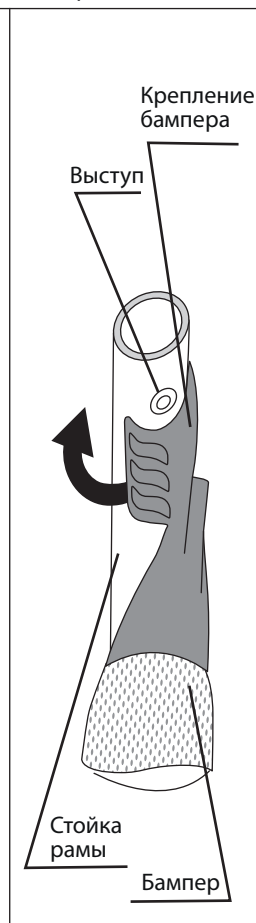
Рис. 4 Крепление бампера
