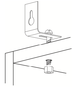
Рис.9 Монтаж навеса
