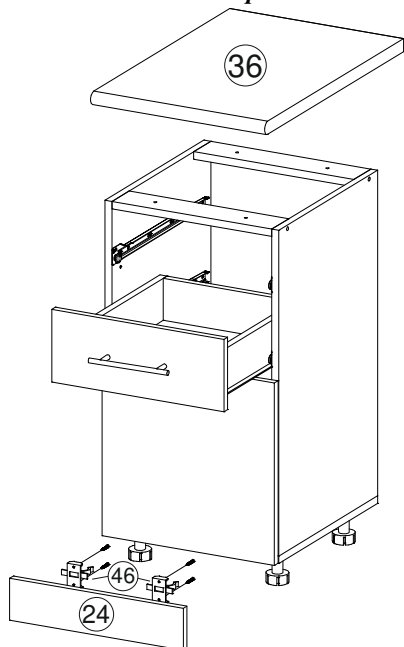
Рис.19 Окончательная сборка
