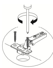
Рис.8 Монтаж чашки петли на фасад
