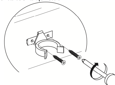
Рис.18 Монтаж клипс и установка цоколя
