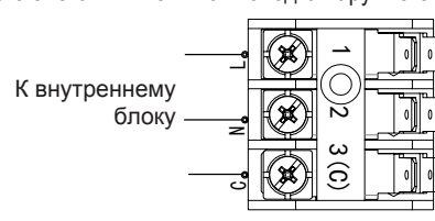
Клеммная колодка наружного блока
