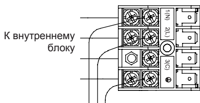
Клеммная колодка наружного блока
