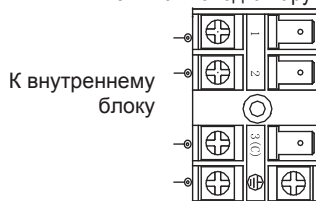
Клеммная колодка наружного блока
