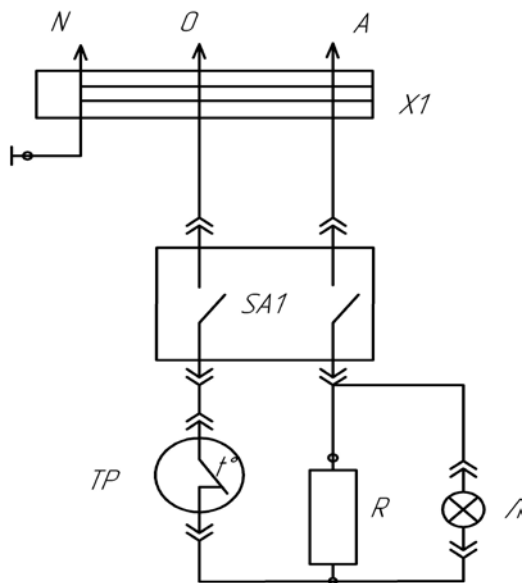
Рис.1 Схема электрическая принципиальная
