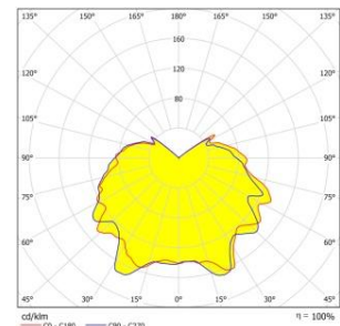
Рисунок 2 – Световое распределение лампы E14 G45 8W.
