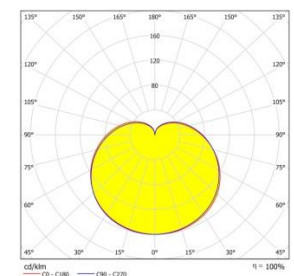
Рисунок 2 – Световое распределение лампы E27 A60 10W.
