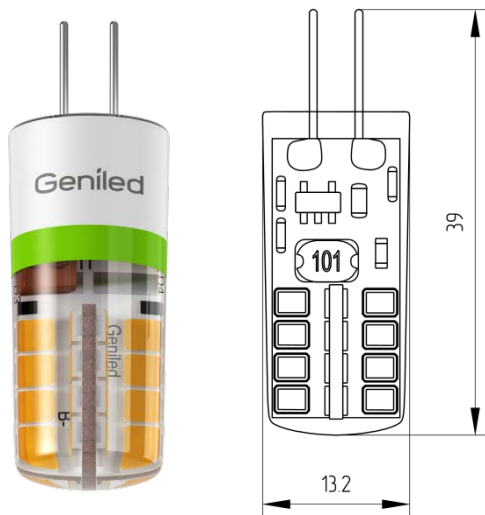
Рисунок 1 – Внешний вид и чертёж.
