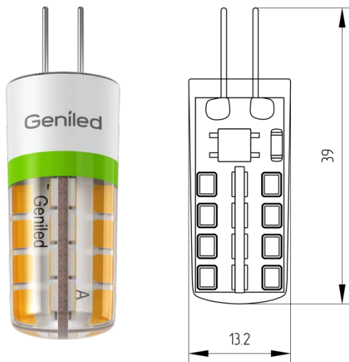
Рисунок 1 – Внешний вид и чертёж.
