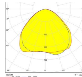
Рисунок 2 – Световое распределение лампы GU5.3 MR16 8W.
