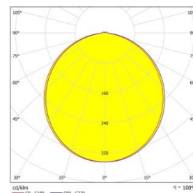
Рисунок 2 – Световое распределение лампы GX53 6W.
