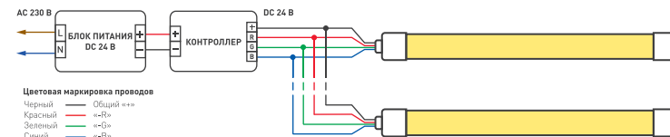
Схема 3. Подключение светодиодных RGB лент NEON.
