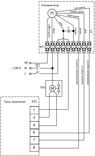
XT1 – XT2 колодка клеммная; YA1 – привод электромагнитного вентилля; QF1 – автоматический выключатель.
