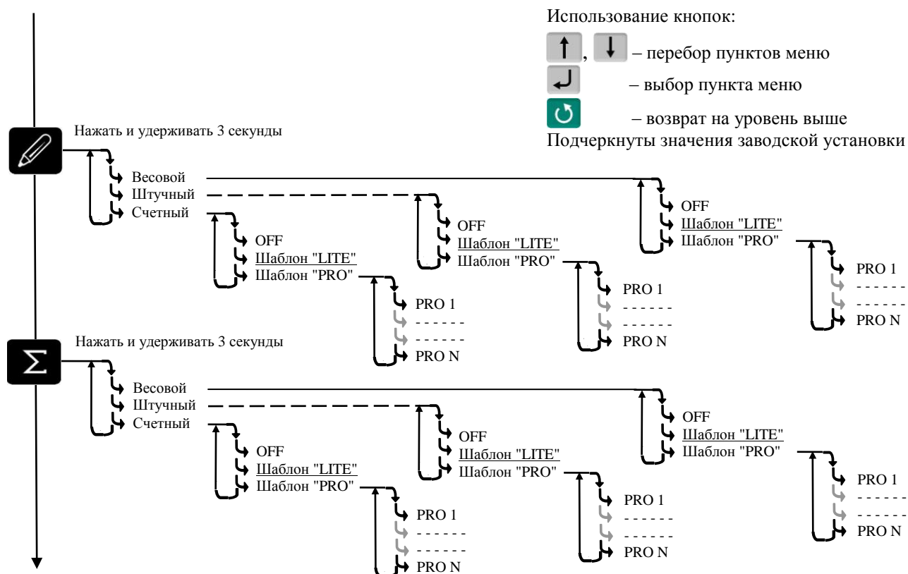
Рис. 4.2 – Схема установки шаблонов печати
