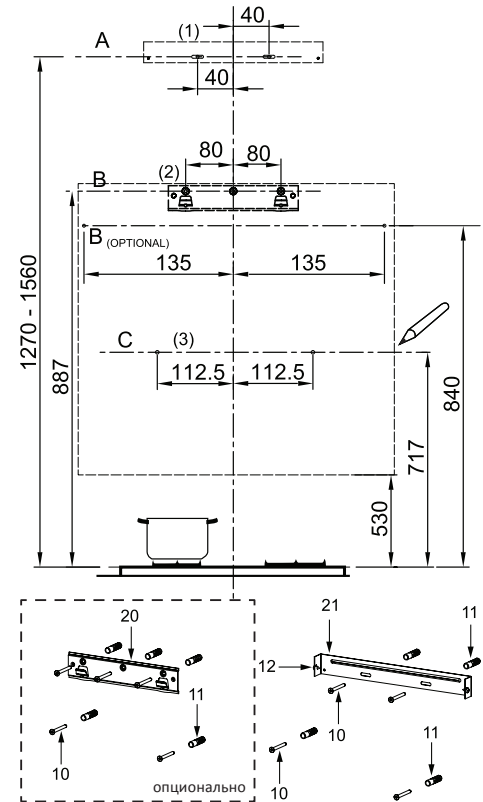
Монтажная схема
