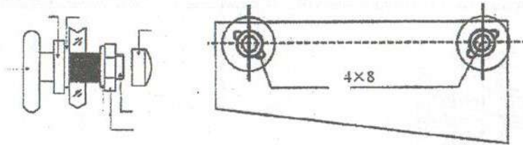
Эксцентрическая ось (конструкция роликов может быть изменена)
