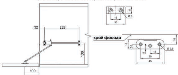
схема крепления барного кранштейна
