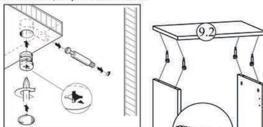
Монтаж эксцентриковой стяжки
