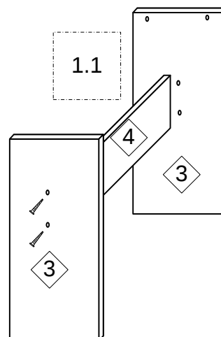
Схема установки стяжки угловой
