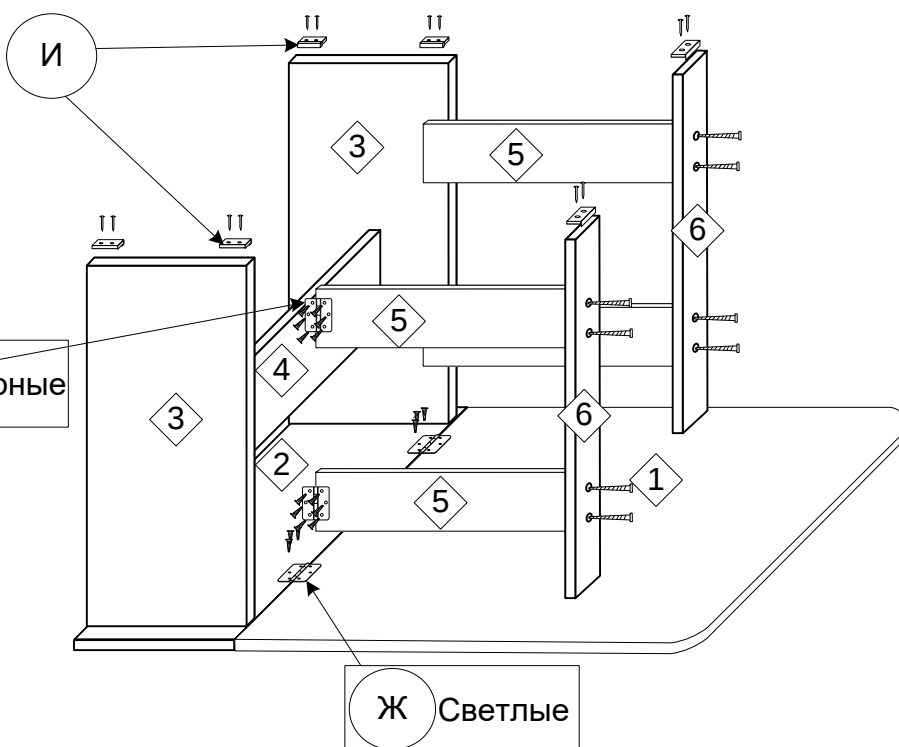
Схема установки опор и столешен
