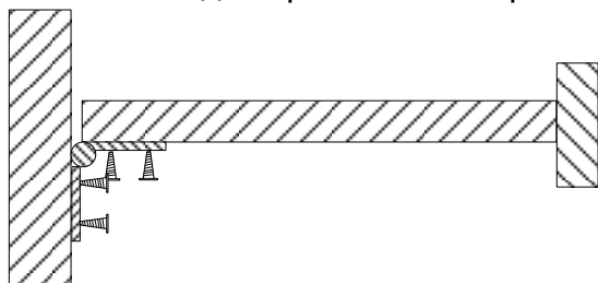
Схема установки петель на боковину для крепления опор
