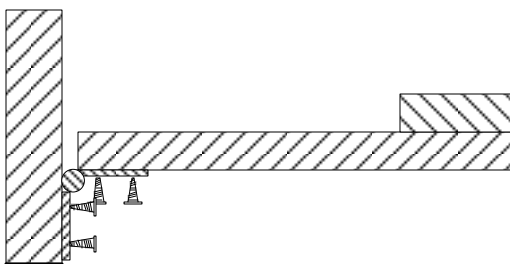
Схема установки петель на боковины для крепления опор
