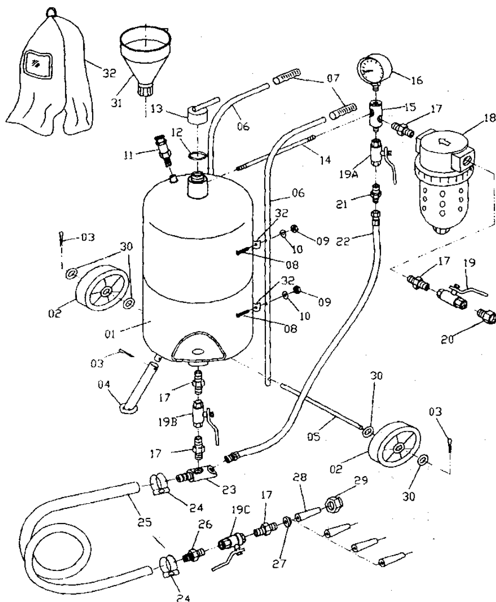
Рис. 1. Устройство изделия.
