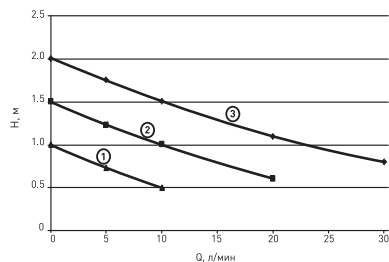
Рабочее поле для насосов CR-25/4, CR-32/4 и CR-25/4-130
