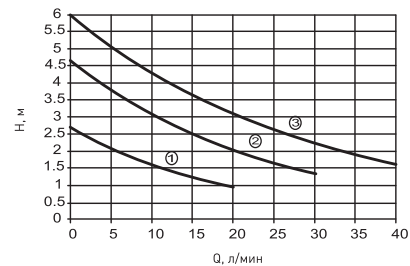
Рабочее поле для насосов CR-25/6, CR-32/6 и CR-25/6-130
