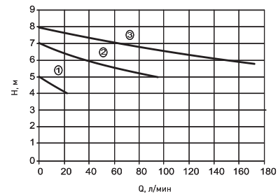
Рабочее поле для насоса CR-32/8
