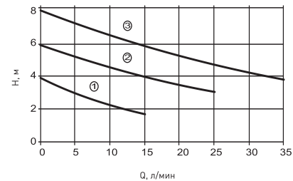
Рабочее поле для насоса CR-25/8
