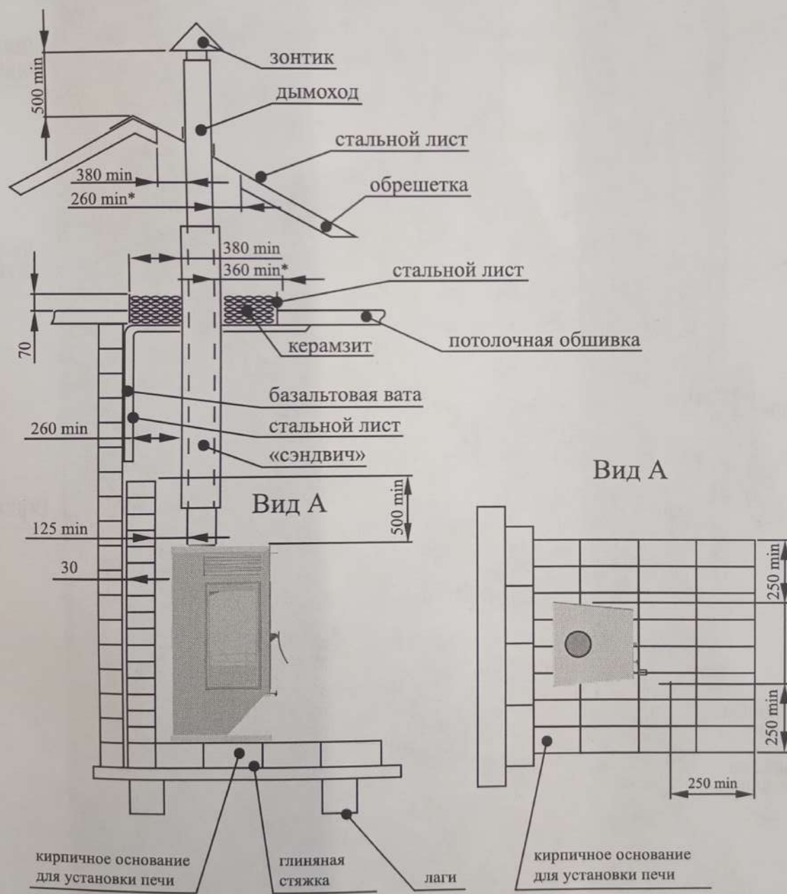
Схема установки печи с расположением дымохода сверху
