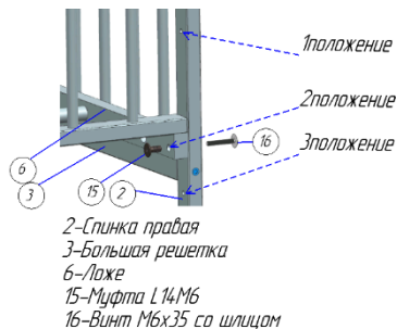
Рисунок 5. Установка Ложье
