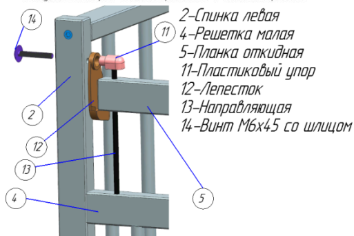
Рисунок 4. Сборка Откидной планки с механизмом опускания «Ушко»
