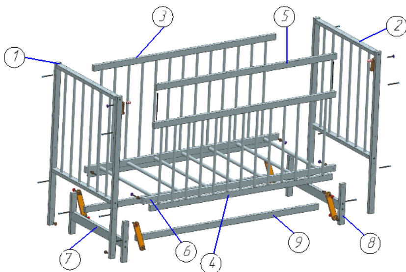
Рисунок1 Основная схема сборки
