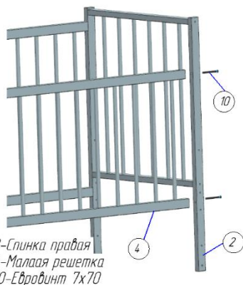
Рисунок 3. Сборка Малой решетки к спинкам кровати
