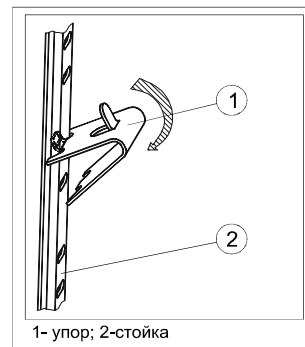
1- упор; 2-стойка
